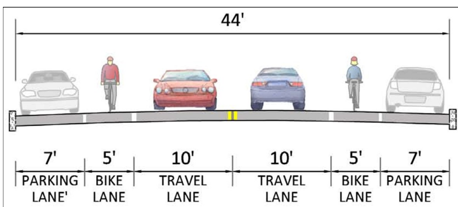
AASHTO Dimensions
