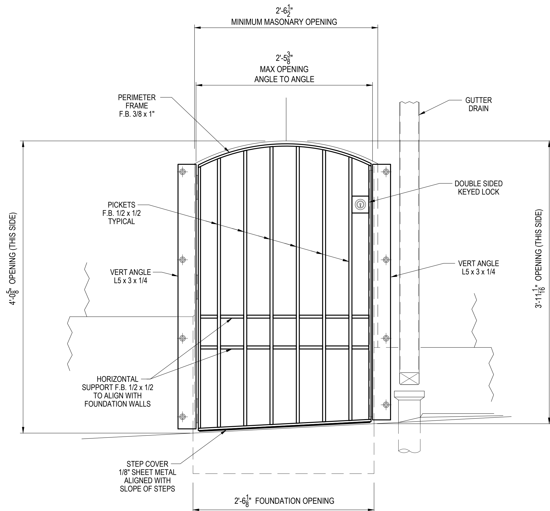
ELEVATION
